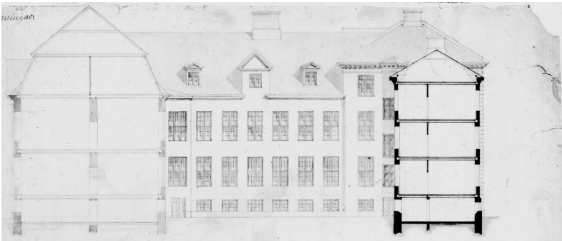
Originaltegning af Frederik Vilhelm Tvede, 1868. Opstalt fra gården, Amaliegade 40. Fra venstre: Snit igennem Jan von Ostens Gård og opstalt af sidehus, Amaliegade 40, herefter opstalt / snit igennem Tvedes baghus / tilbygning.
